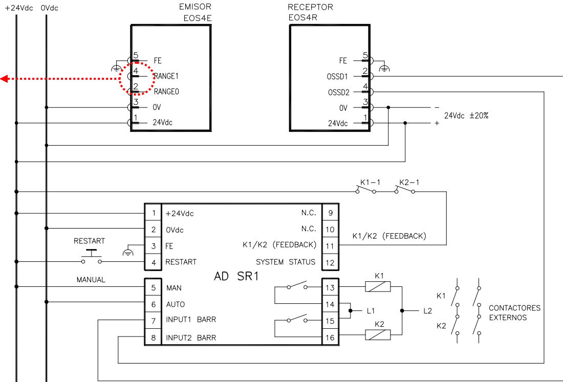
Figura 21 - EOS4 A: Funcionamiento manual con módulo ADSR1
