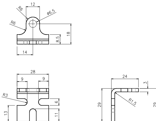
Figura 30 - Escuadras de fijación SFB180E
