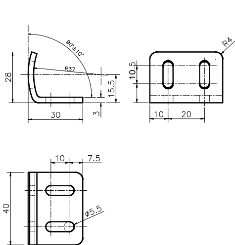
Figura 29 - Escuadras de fijación SFBE
