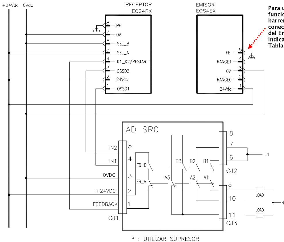
Figura 22 - EOS4 X: Funcionamiento automático con módulo ADSR0
