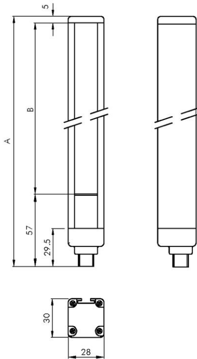
EOS4 A - EOS4 X - EOS4 Slave (Emisor y Receptor)
