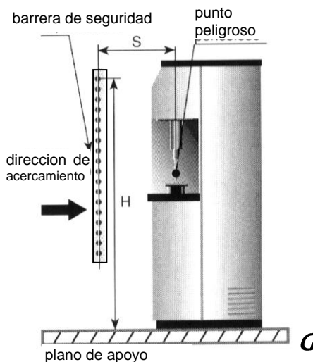
Figura 12 - Ubicación vertical 14mm, 20mm, 30mm, 40mm
